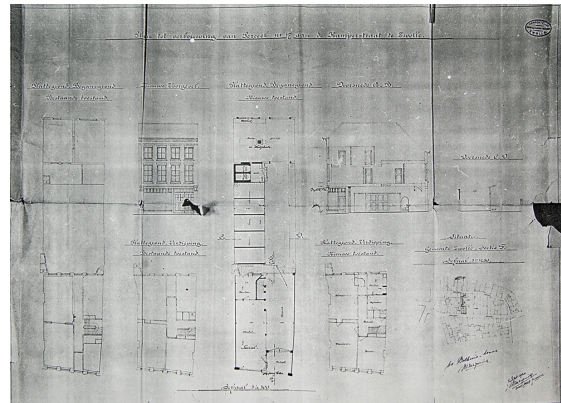
Verbouwings-tekening door architect M. Meijerink uit 1920 van de verbouwing tot autobedrijf.
