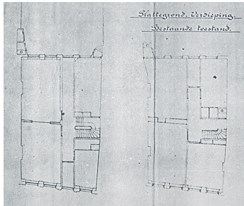
Bestaande toestand van een verbouwingstekening uit 1920 die de in de 19e eeuw ontstane indeling goed weergeeft.
