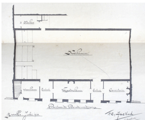
Opmeting van de begane grond van het kerkgebouw uit 1910. De weergegeven situatie zal in grote lijn in 1846 ontstaan zijn. [HCO]
