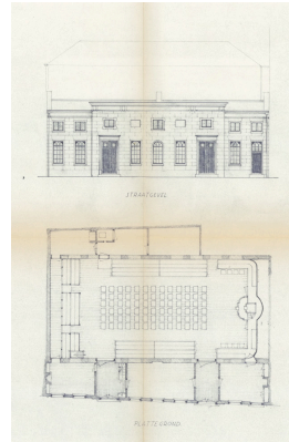
Opmeting van de voorgevel en plattegrond uit 1969. [HCO]
