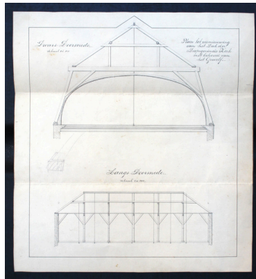
Plantekening van een nieuwe kap over de kerkruijnte. Deze tekening betreft een niet uitgevoerde variant, waarbij het bestaande gewelfde plafond gehandhaafd zou worden. [HCO]
